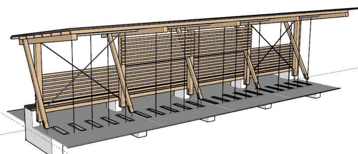
3D-Darstellung der Konstruktion (Bild)
