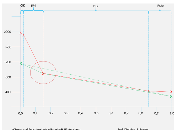
Wärme- und Feuchteschutz – Bauphysik HS Augsburg Prof. Dipl.-Ing. S. Runkel Dampfdiffusionsverlauf - Tauwasser (Quelle eigene Darstellung)
